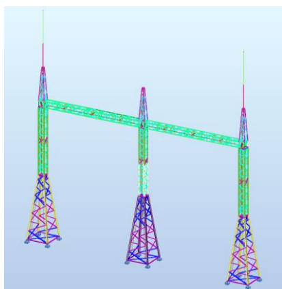
110 kV Linijinis portalas
