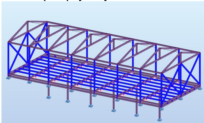
Valdymo pulto pastato antžeminės dalies konstrukcija
